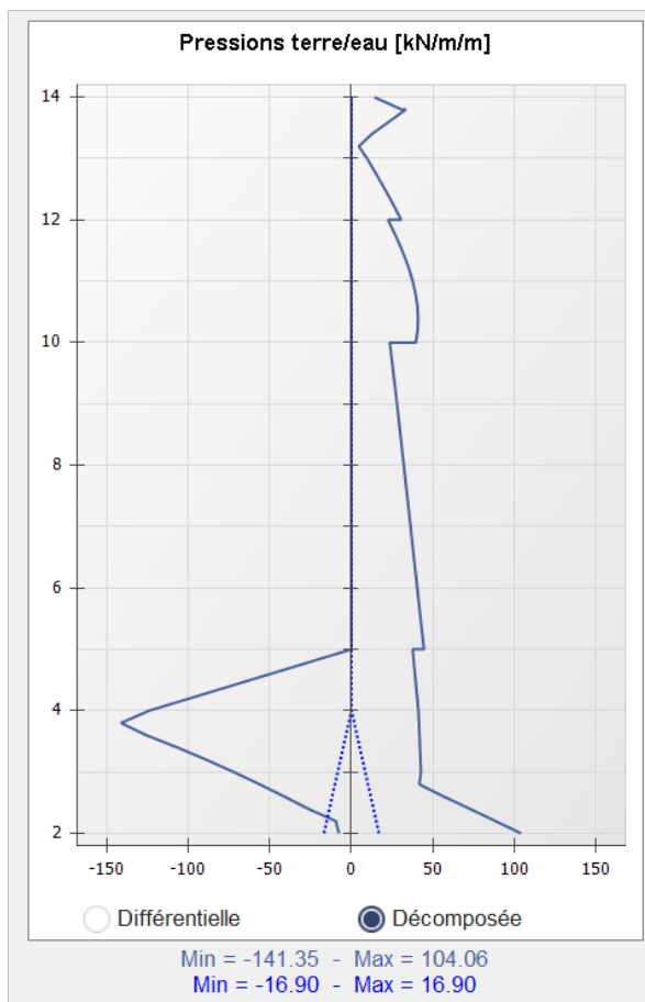
Profils de pressions avant diminution de p_{\max}
