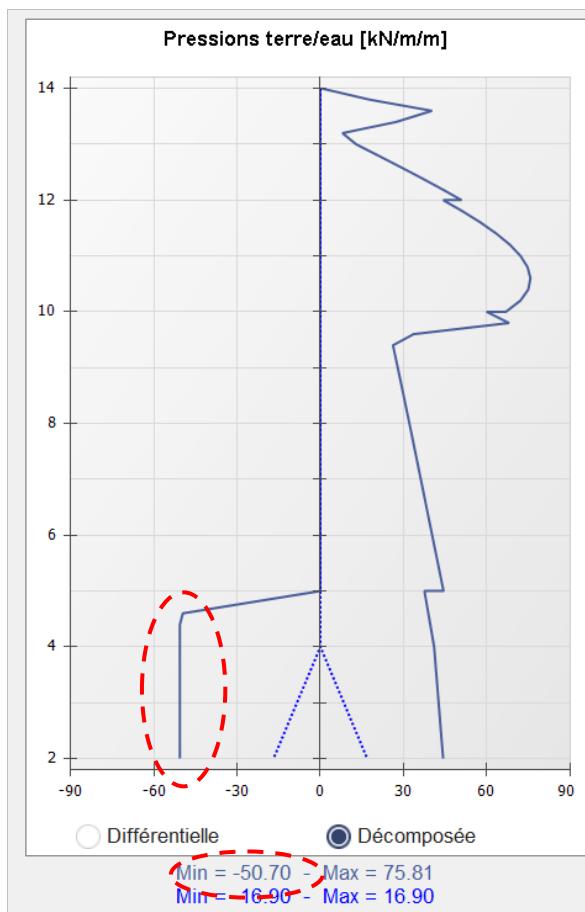
Profils de pressions après diminution de p_{\max}
